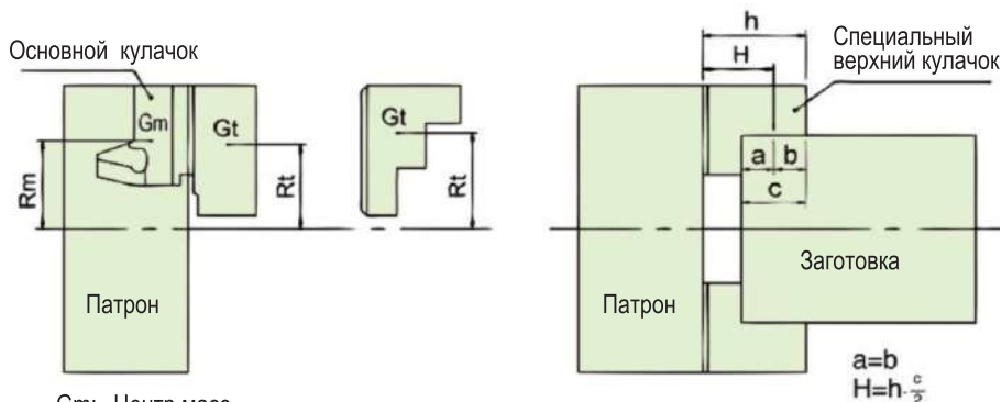
Рисунок 2. Специальный верхний кулачок
